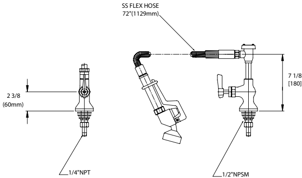
KL63-2000-VB shown
